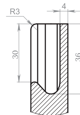
Вид ручки в разрезе
